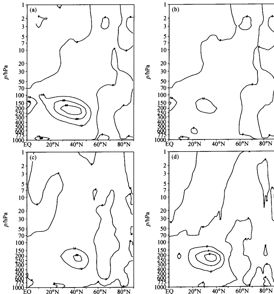
图 2 同图 1, 但为夏季
