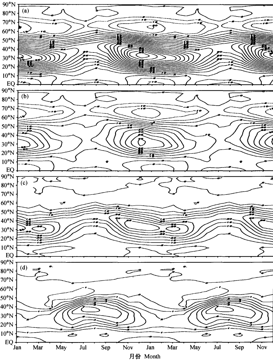
图 5 250 hPa 等压面上气候平均的不同尺度定常波对动量输送的逐月变化 (单位: m^2/s^2 ): (a) 总波动; (b) 行星尺度 (1~3) 波; (c) 天气尺度 (4~9) 波; (d) 10 波以上短波
