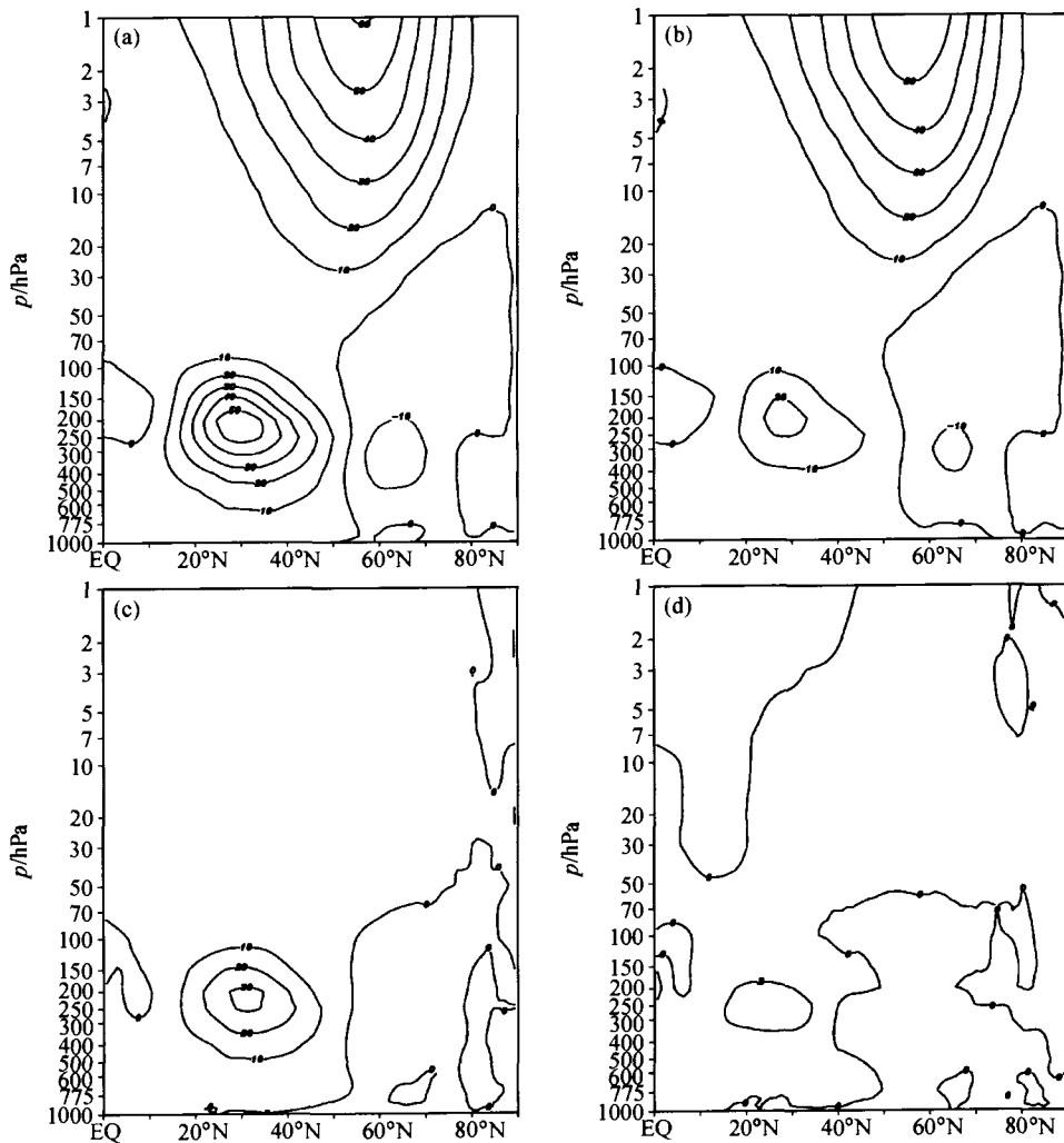
图1 春季纬向平均状态下不同尺度定常波对西风动量输送的纬度-高度剖面图（单位：m 2 /s 2 ）：(a) 总波动；(b) 行星尺度(1~3)波；(c) 天气尺度(4~9)波；(d) 10波以上的短波。向北通量为正，向南通量为负
