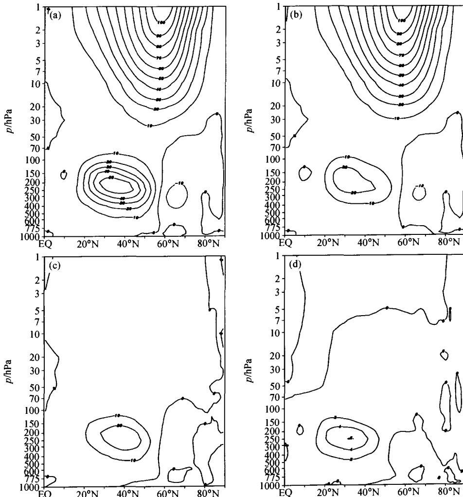
图 3 同图 1, 但为秋季
