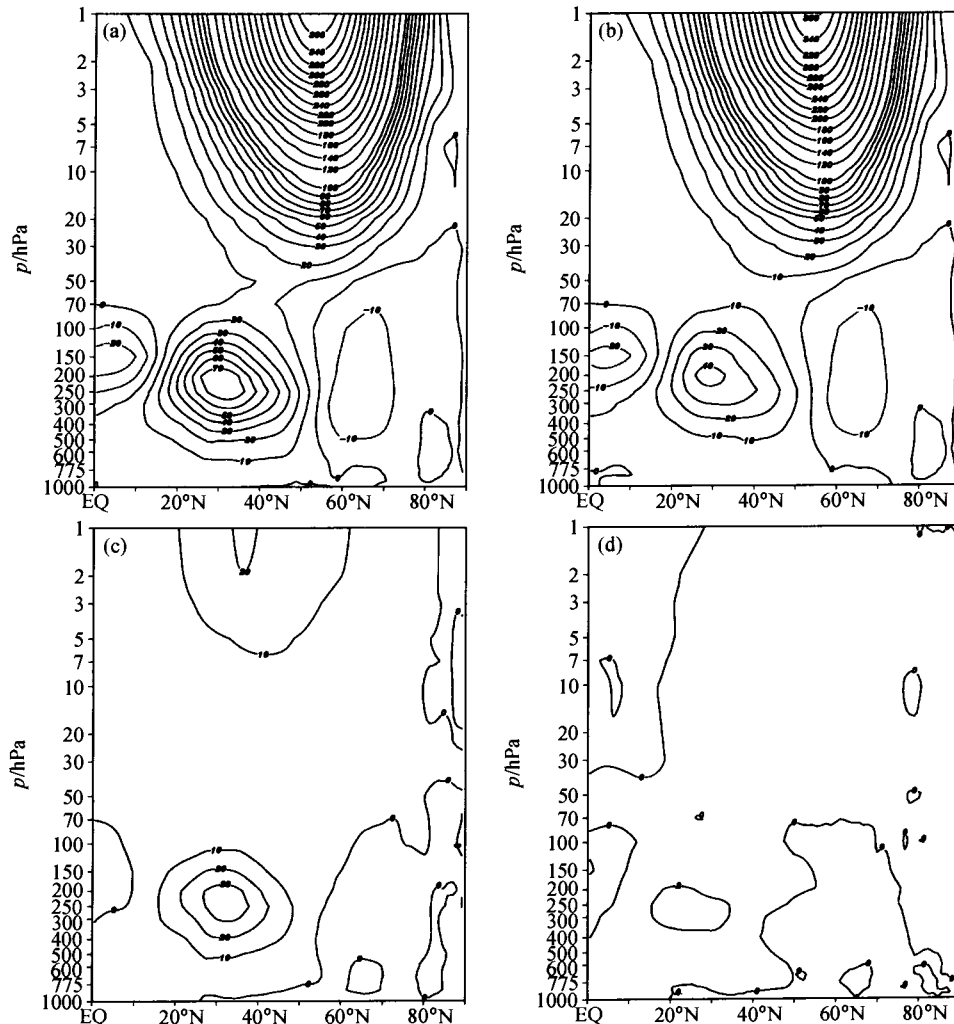
图 4 同图 1, 但为冬季 Fig. 4 Same as Fig. 1, but for winter
