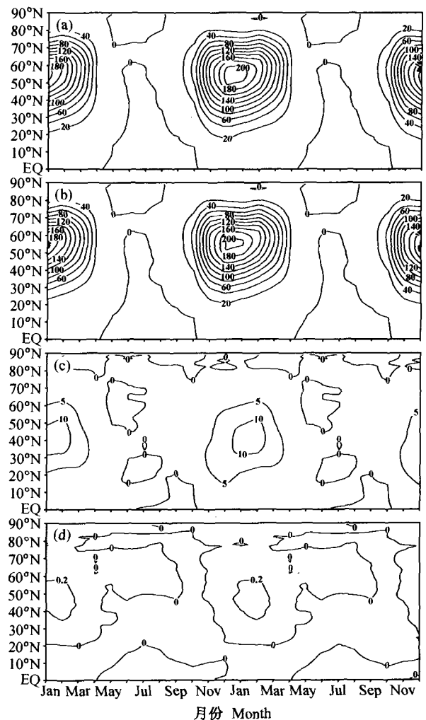
图 6 同图 5, 但为 5 hPa 等压面
